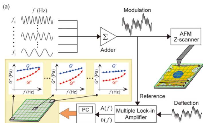
図1 多重周波数フォースモジュレーション法の概念図。複数個（ n 個）の周波数信号を重畳した励振信号をカンチレバーに印加し、1回の押し込み測定における細胞変形の周波数応答を多重ロックインアンプより検波し、その測定点における細胞の複素弾性率の周波数特性を測定する。
